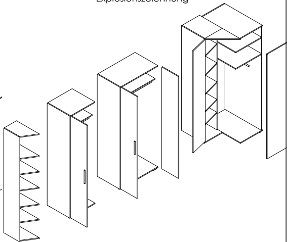
Explosionszeichnung
