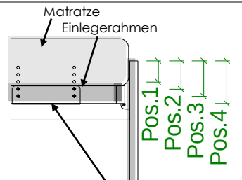
Bsp. zeigt Rahmenauflage auf Pos.4
