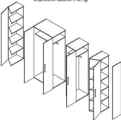
Explosionszeichnung
