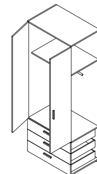
z Grundelement 2-türig mit 3 Schubkästen 90 cm
