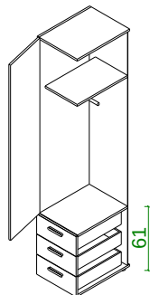
z Grundelement 1-türig mit 3 Schubkästen 45 cm
